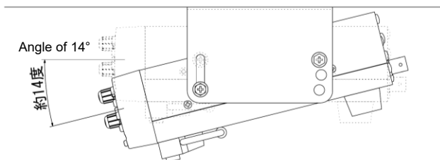
ブラケットを上側に取り付けた場合
