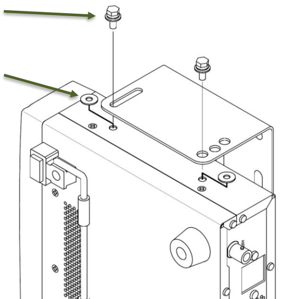
受信機の取り付け図
