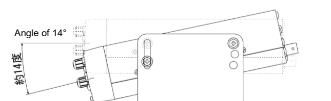
ブラケットを下側に取り付けた場合
